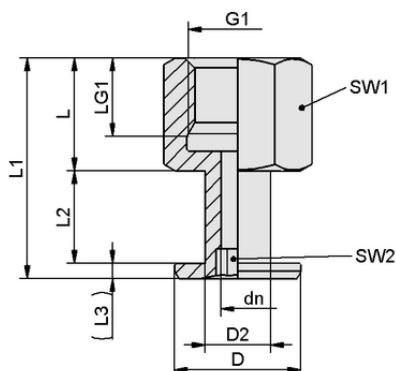
Конструктивные данные SA-NIP N006 G1/8-IG DN200
