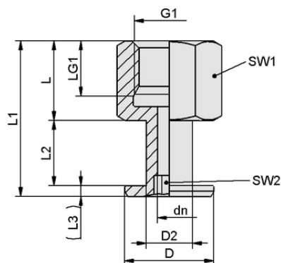
Конструктивные данные SA-NIP N004 G1/8-IG DN200
