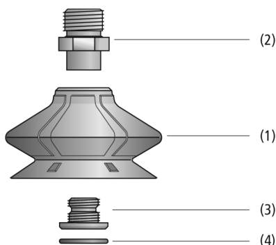
Конструкция системы Сильфонные присоски SPB1 (1,5 гофра, Одиночный компонент)
