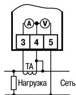
Рисунок 5.3 – Подключение прибора к однофазной сети через согласующий трансформатор тока
