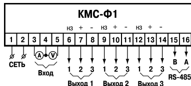
Рисунок 5.1 – Назначение клеммника
