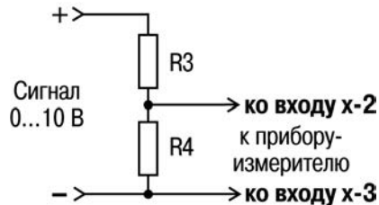
Рисунок 3.1 – Электрическая схема делителя (R3=1800,0 Ом, R4=200,0 Ом)
