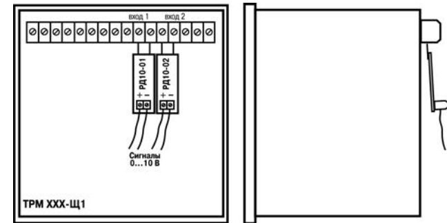
Рисунок 3.2 – Подключение делителей к двухканальному ТРМ в корпусе Щ1
