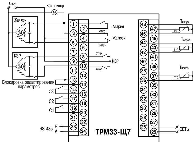
Рисунок В.3 – Схема подключения TPM33-Щ7
