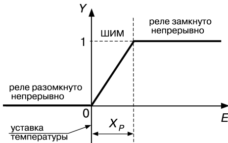
Рис. 3.7. П-закон регулирования
