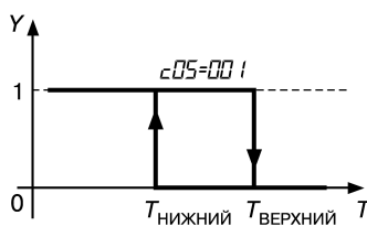
Рис. 3.15. Компаратор срабатывает по нижней уставке:
