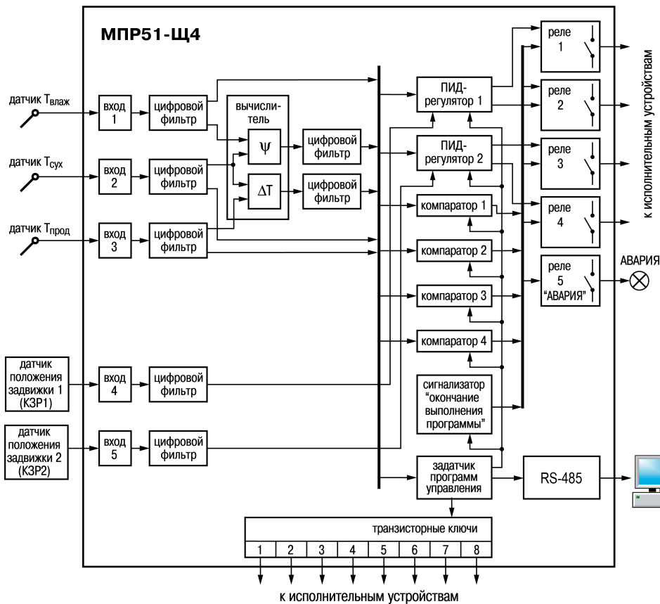
Рисунок 3.1. Структурная схема
