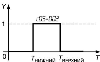
Рис. 3.16. Компаратор срабатывает внутри установленных пределов
