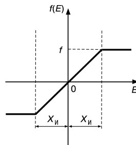
Рис. 3.9. Ограничение интегральной составляющей при помощи X_{\text{и}}
