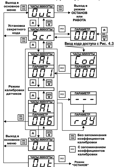
Рис. 4.6. Схема, поясняющая работу на уровне L4
