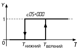
Рис. 3.14. Компаратор срабатывает по верхней уставке:
