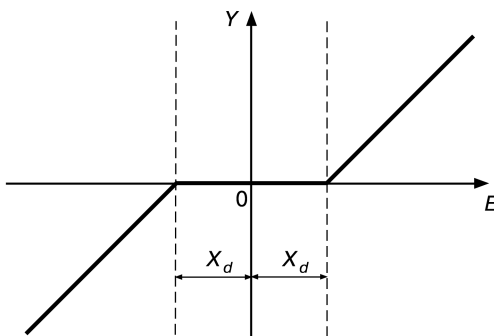
Рис. 3.13. Зона нечувствительности для исполнительного устройства типа "нагреватель - холодильник" или "завдвижка"
