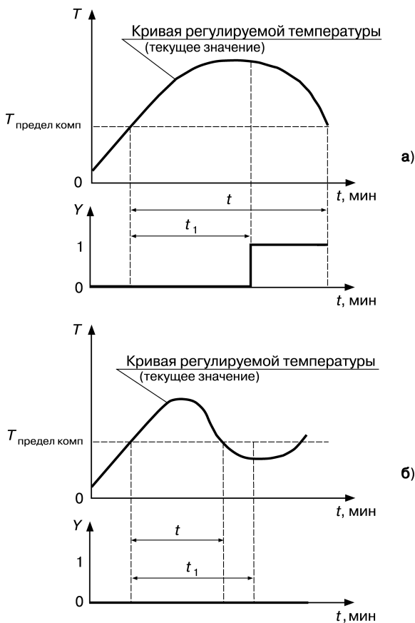
Рис. 3.19. Задержка срабатывания компаратора:
