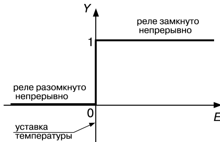
Рис. 3.8. Т-закон регулирования (релейный): полоса пропорциональности X_p равна нулю
