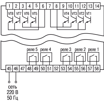
Рис. Б.2. Подключение транзисторных ключей и выходных устройств
