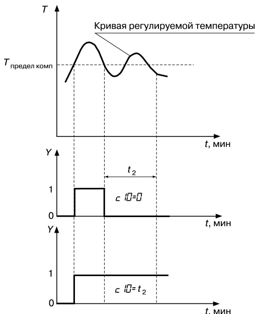
Рис. 3.20. Задержка отпущения компаратора: компаратор "не отпустил"
