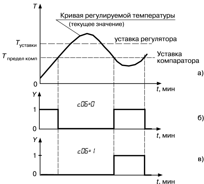
Рис. 3.18. Блокировка срабатывания компаратора до 1-го достижения уставки
