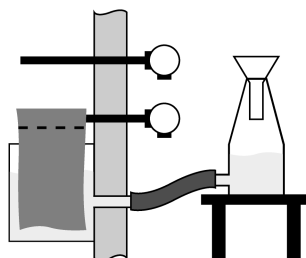
Рис. Е.4. Конструкция резервуара для воды, не требующая входа в камеру
