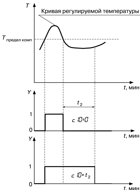
Рис. 3.21. Задержка отпущения компаратора: компаратор "отпустил"
