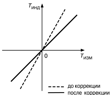
Рис. 3.6. Коррекция "наклон характеристики"
