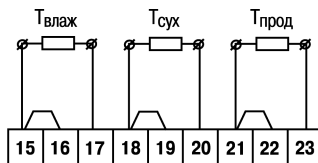
Рис. В.2. Соединение датчиков по двухпроводной схеме
