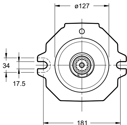
SAE C, 2 отверстия для HPR 55, 75, 105
