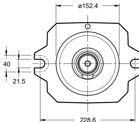
SAE D, 2 отверстия для HPR 135
